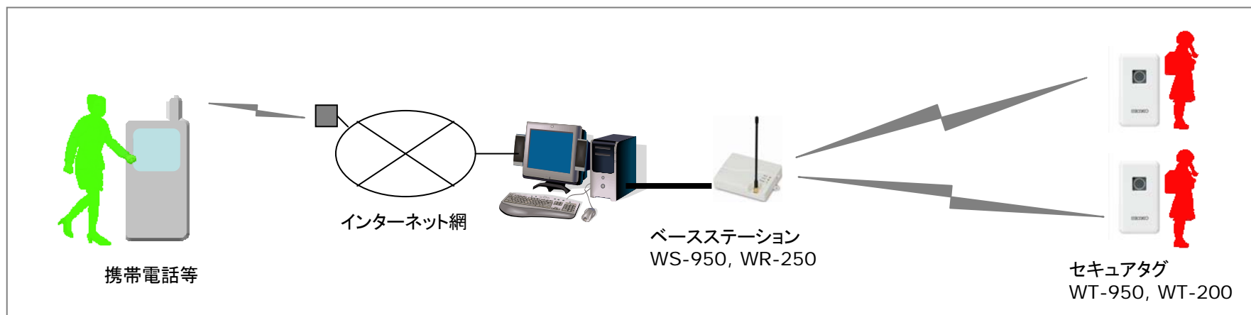
〈図1-1〉児童見守りシステム基本動作
