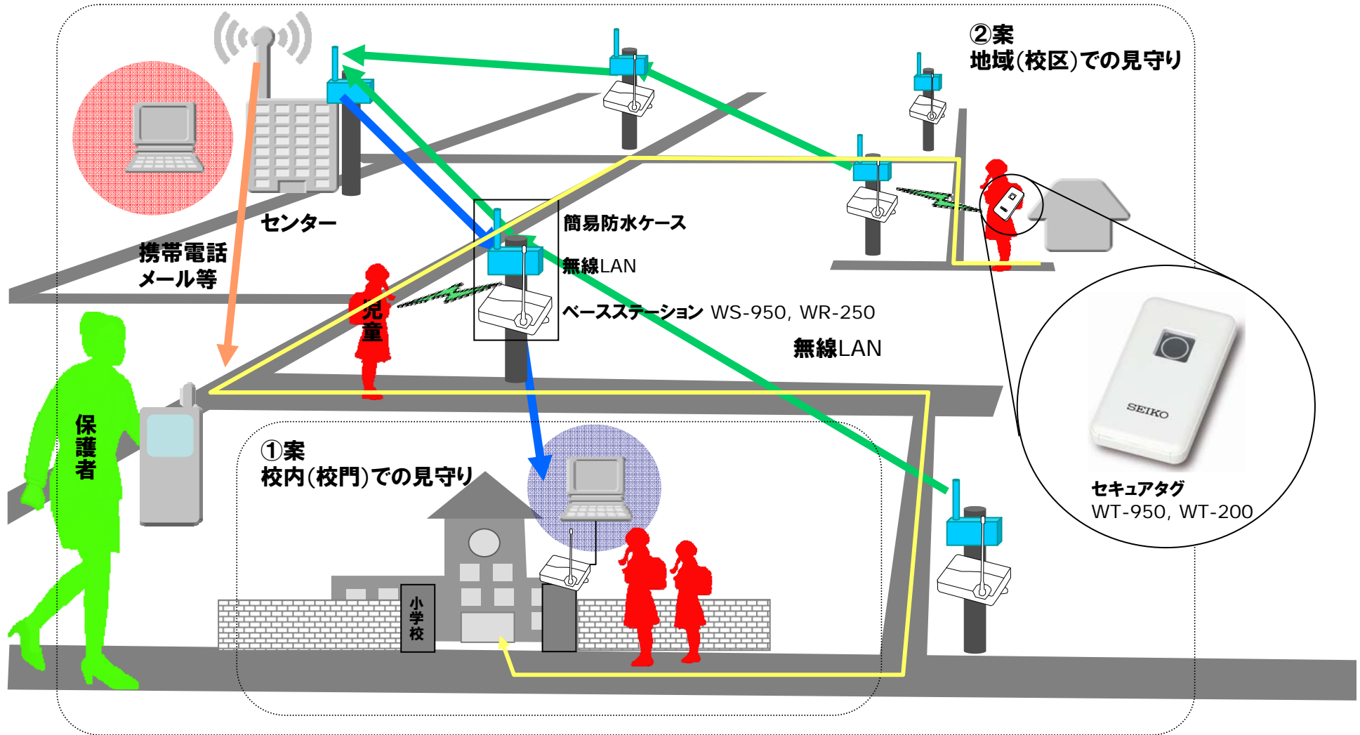
<図1-2>児童見守りシステムイメージ図
