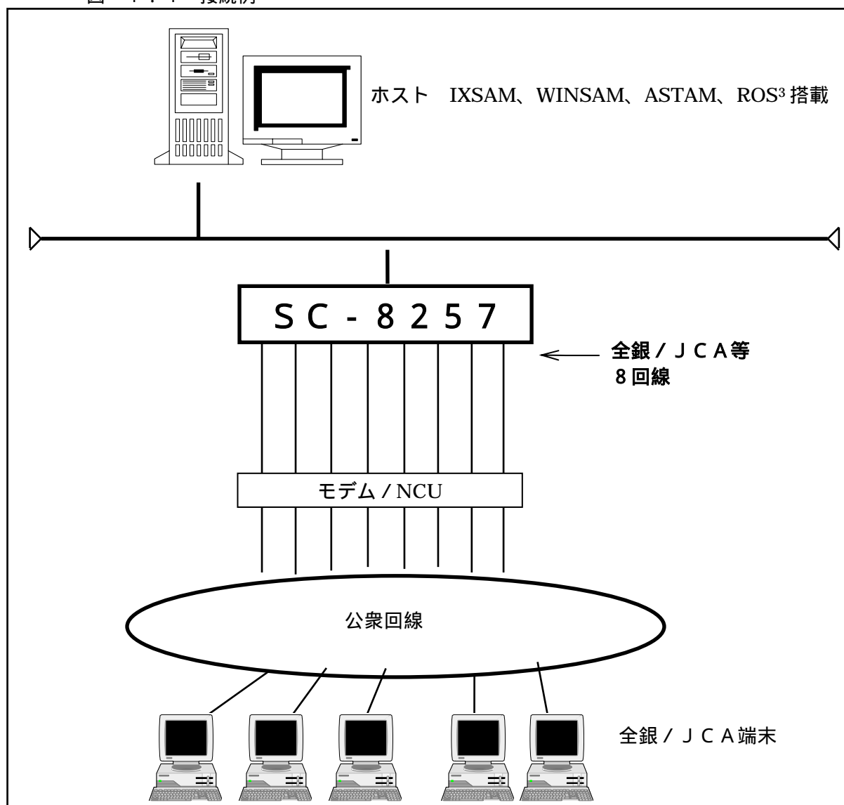
図 1.4 接続例
