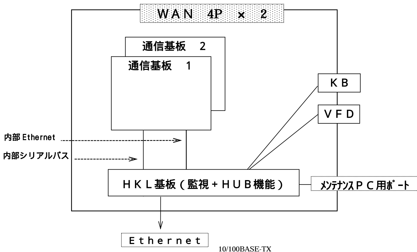
図 1.5 SC-8257構成
