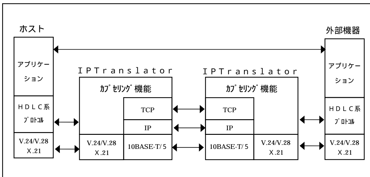
図 1.2 プロトコル構成
